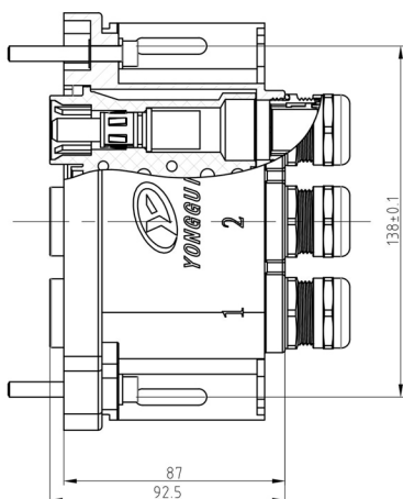
插头外形尺寸：
