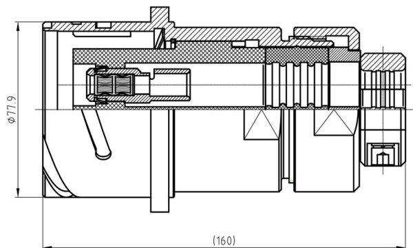
插座外形尺寸：
