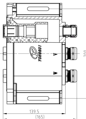
插座外形尺寸：
