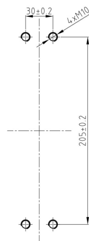
安装开孔尺寸：
