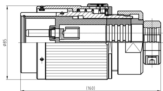
插头外形尺寸：
