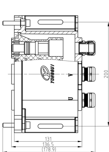
插头外形尺寸：
