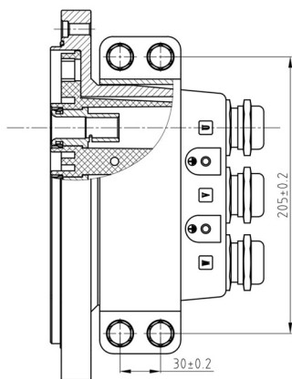
插座外形尺寸：
