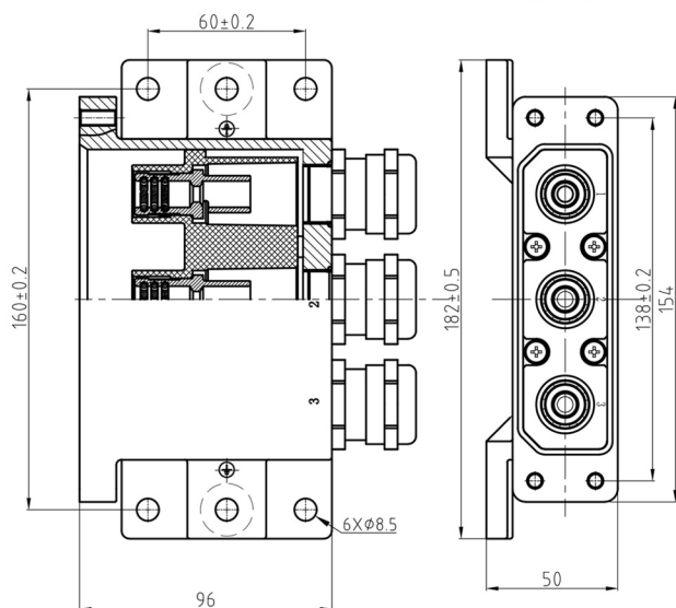
插座外形尺寸：
