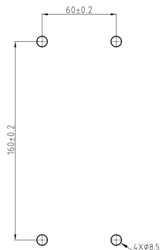
安装开孔尺寸：
