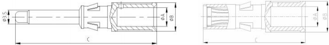
Φ3.5针孔尺寸示意图Socket dimension diagram
