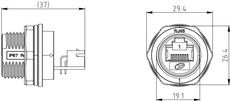
插座装配防水盖组件后外形图示
