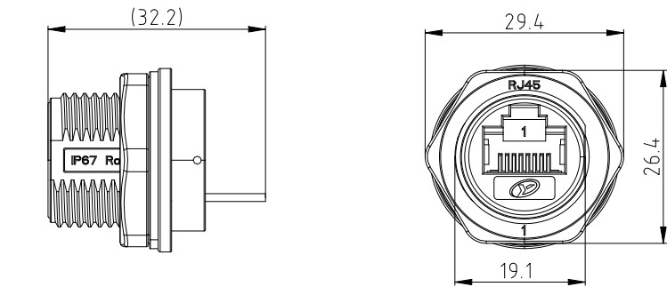
插座装配防护盖组件后外形图示
