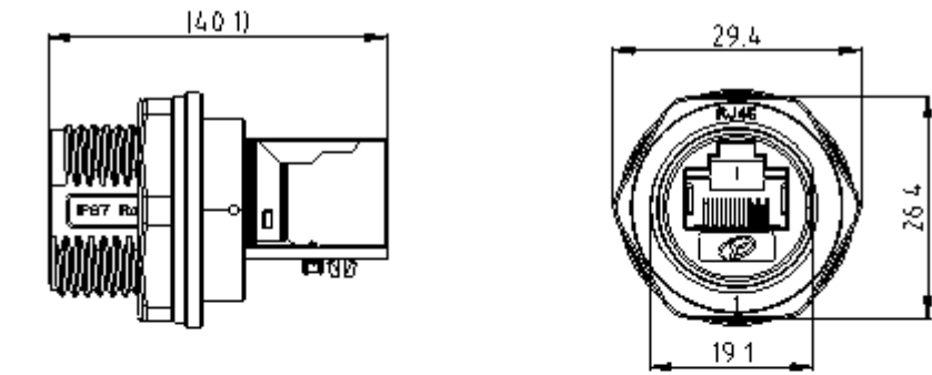
插座装配防护盖组件后外形图示
