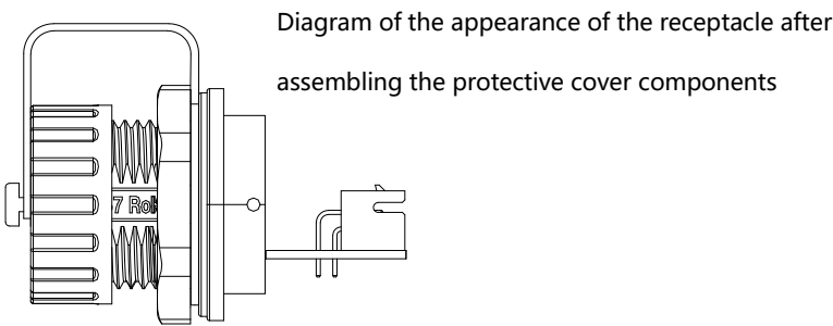
插座装配防水盖组件后外形图示
