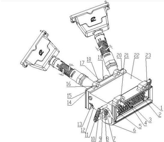
图 1. 电气车钩
