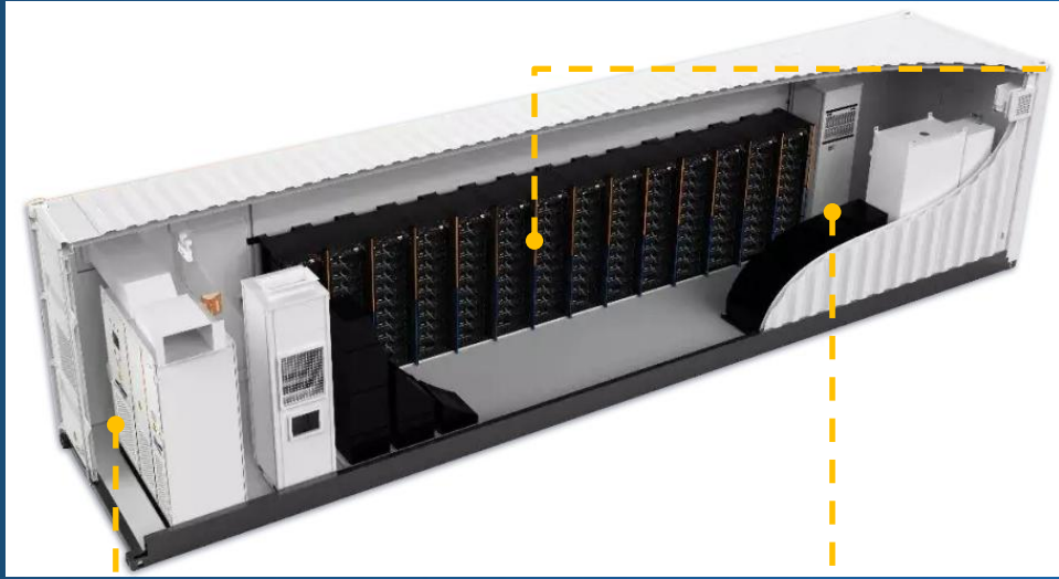
PCS
